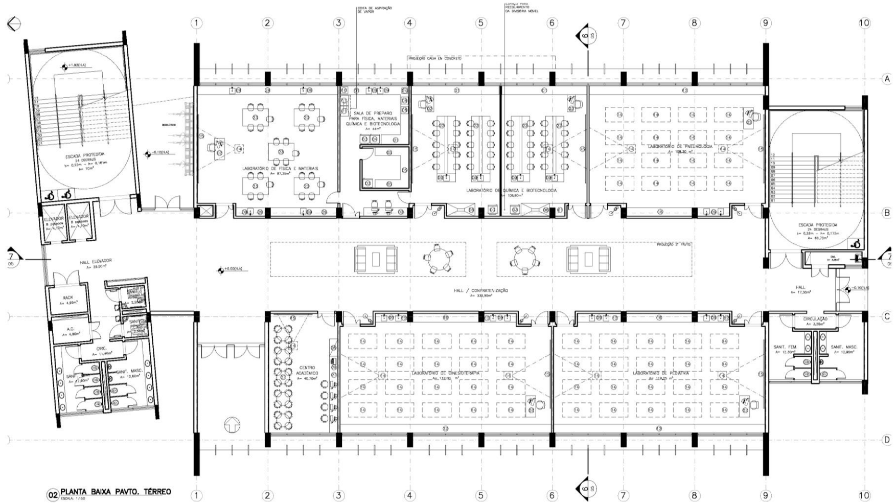
Figura 9 – Planta Baixa do Pavimento térreo do prédio I para o Campus Araranguá.
